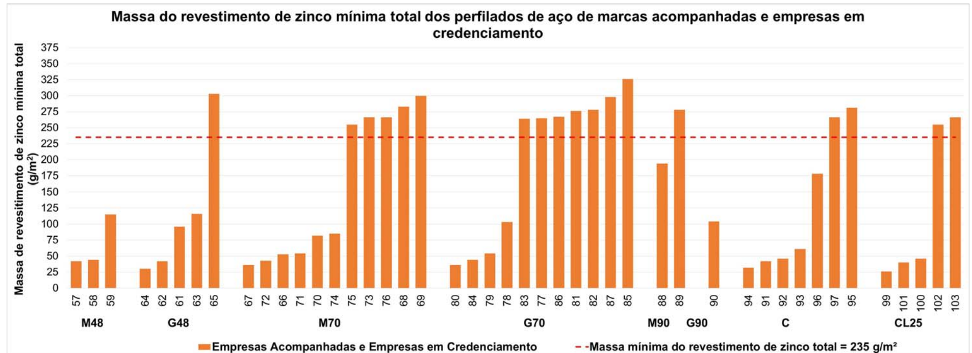
Figura 22 – Resultados da determinação da massa do revestimento de zinco total (nas duas faces) das amostras de perfilados de aço de marcas acompanhadas e em credenciamento avaliadas
