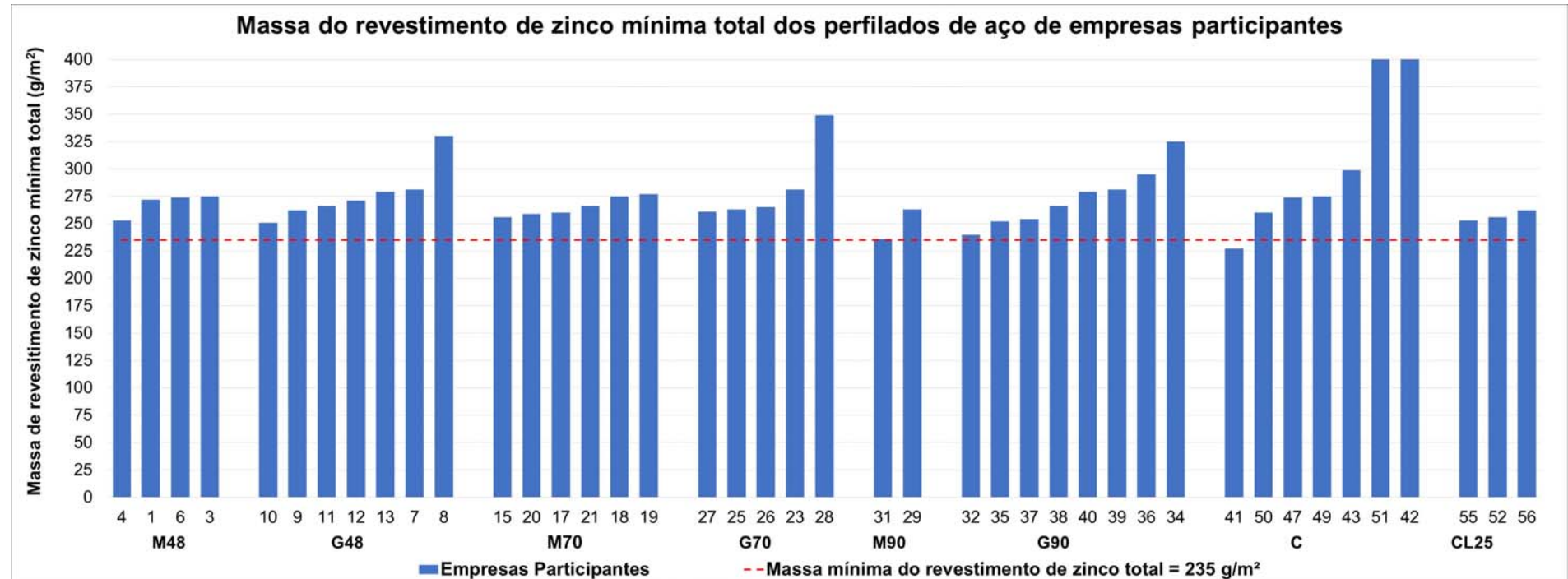
Figura 20 – Resultados da determinação da massa do revestimento de zinco total (nas duas faces) das amostras de perfilados de aço de empresas participantes avaliadas
