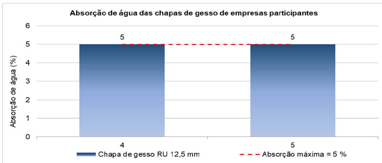
Figura 16 – Resultados da absorção de água de chapas de gesso RU 12,5 mm avaliadas
