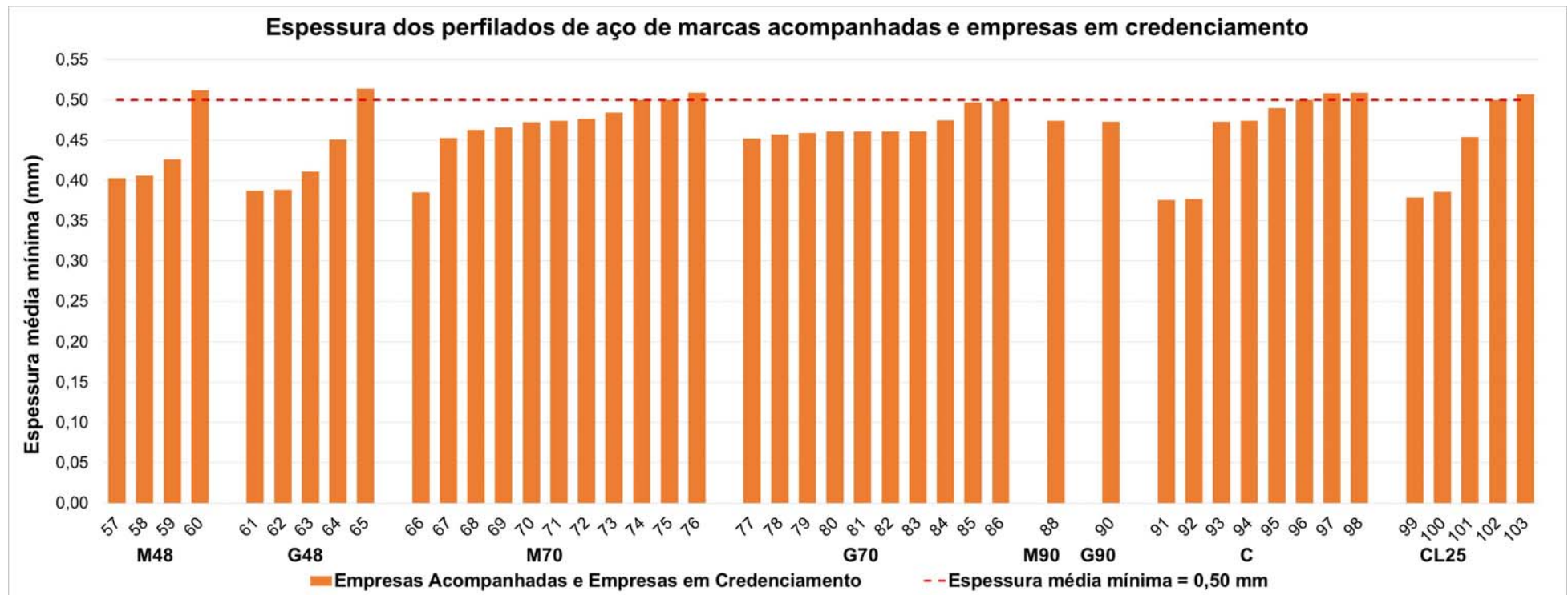
Figura 18 – Resultados da determinação da espessura das amostras de perfilados de aço de marcas acompanhadas e empresas em credenciamento avaliadas
