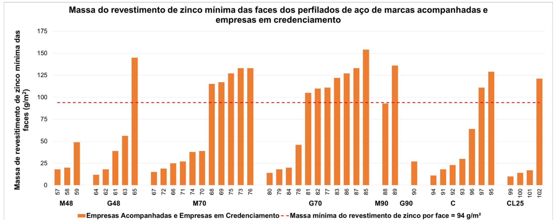
Figura 21 – Resultados da determinação da massa do revestimento de zinco mínima das faces das amostras de perfilados de aço de marcas acompanhadas e em credenciamento avaliadas
