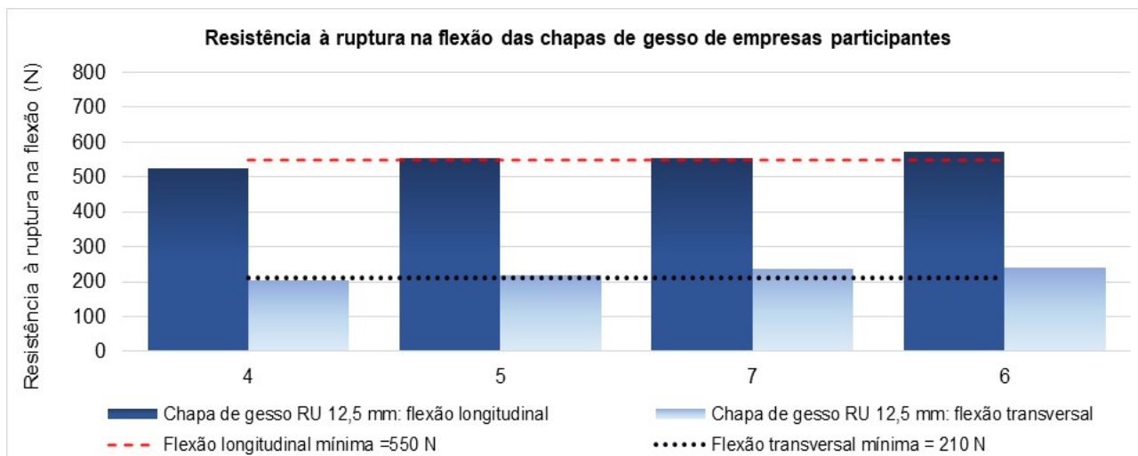
Figura 15 – Resultados da determinação da resistência à flexão (média) das amostras de chapas de gesso RU 12,5 mm avaliadas
