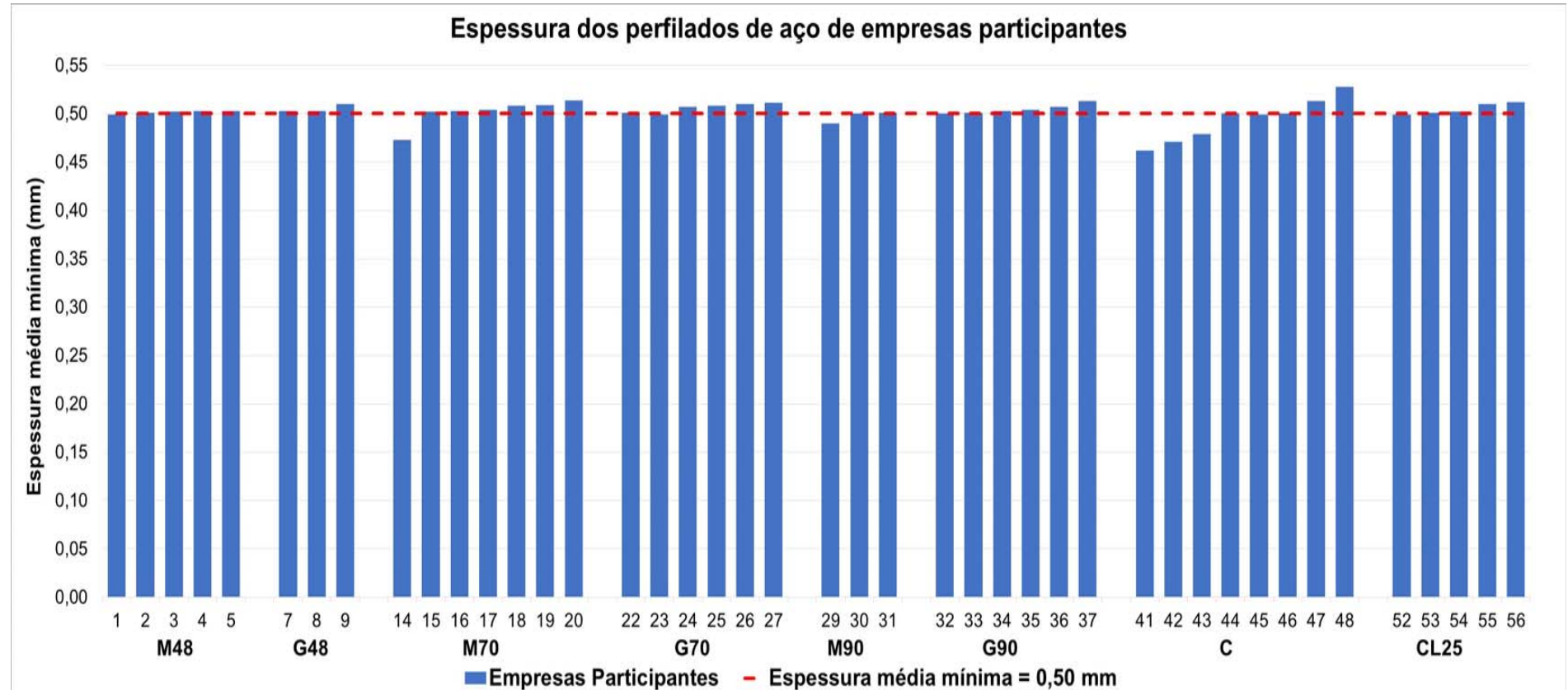
Figura 17 – Resultados da determinação da espessura das amostras de perfilados de aço de empresas participantes avaliadas
