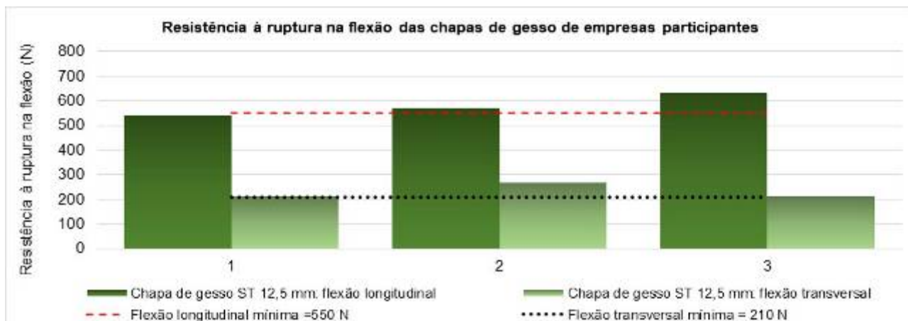
Figura 13 – Resultados da determinação da resistência à flexão (média) das amostras de chapas de gesso ST 12,5 mm avaliadas
