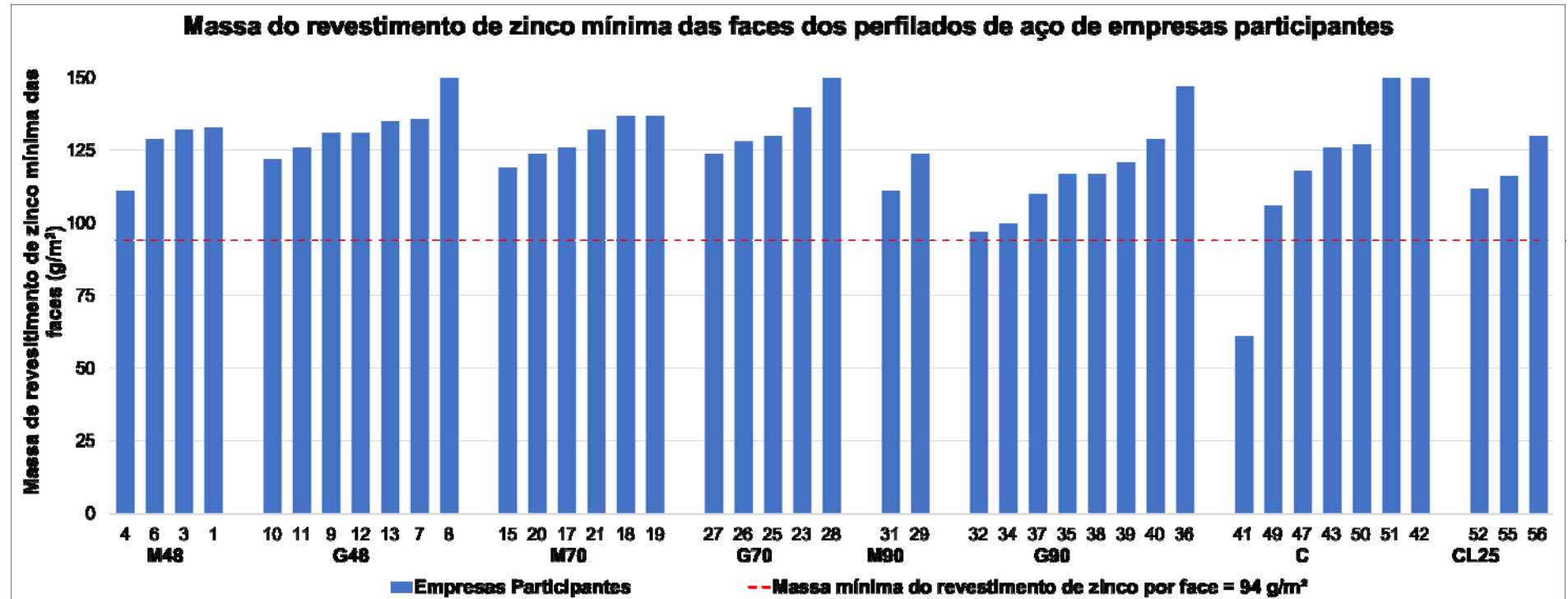
Figura 19 – Resultados da determinação da massa do revestimento de zinco mínima das faces das amostras de perfilados de aço de empresas participantes avaliadas
