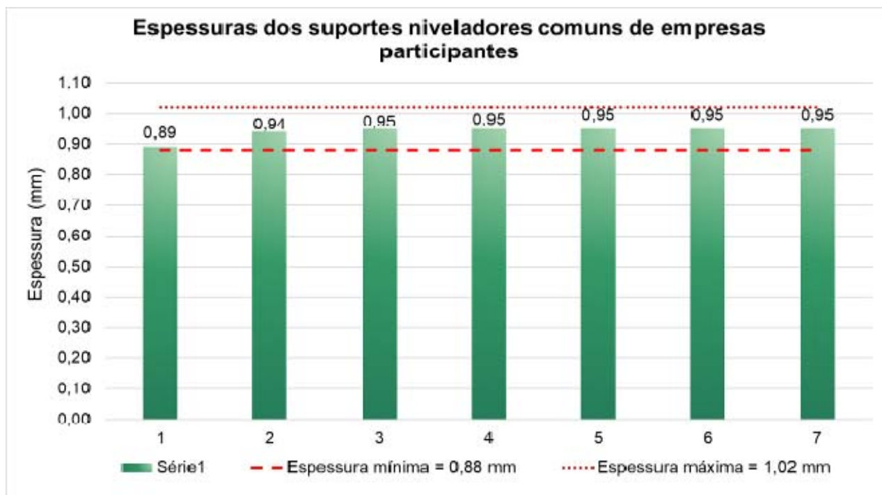
Figura 23 – Resultados da determinação da espessura das amostras de suporte nivelador comum avaliadas de empresas participantes
