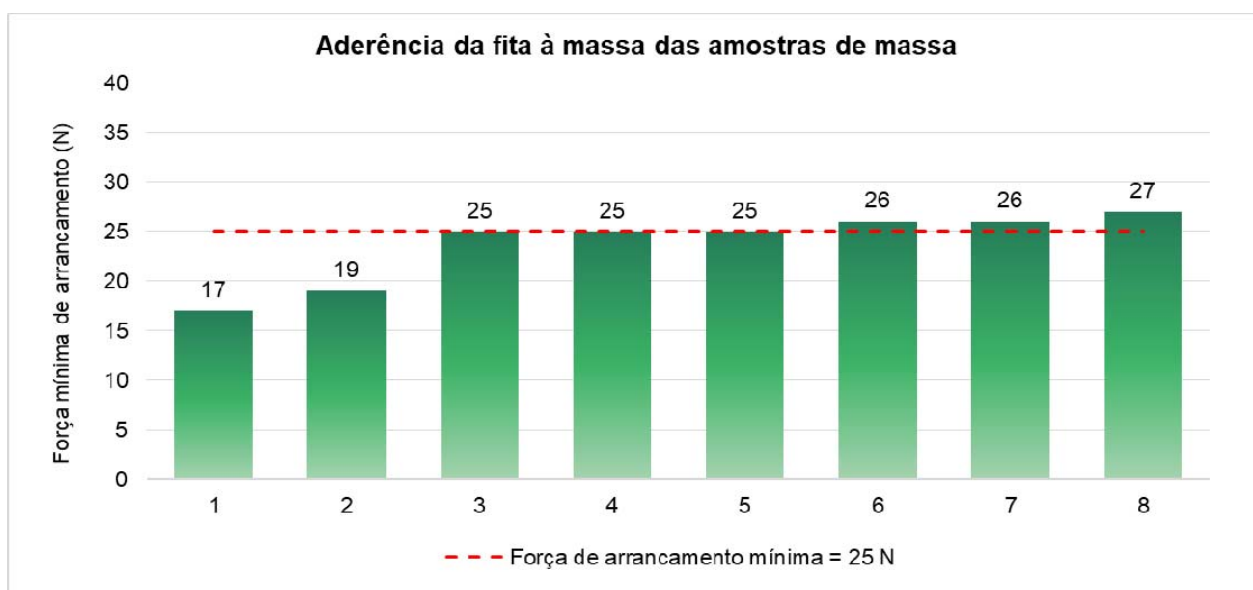
Figura 26 – Resultados da verificação da aderência da fita à massa das amostras de massa para tratamento de juntas avaliadas (empresas participantes e marca acompanhada)
