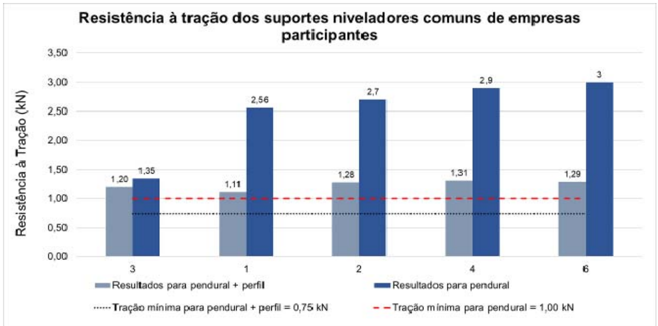
Figura 24 – Resultados da determinação resistência à tração das amostras de suporte nivelador comum avaliadas de empresas participantes
