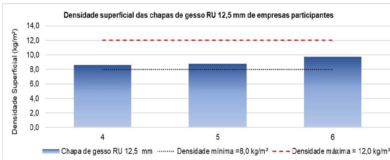
Figura 14 – Resultados da determinação da densidade superficial das amostras de chapas de gesso RU 12,5 mm avaliadas
