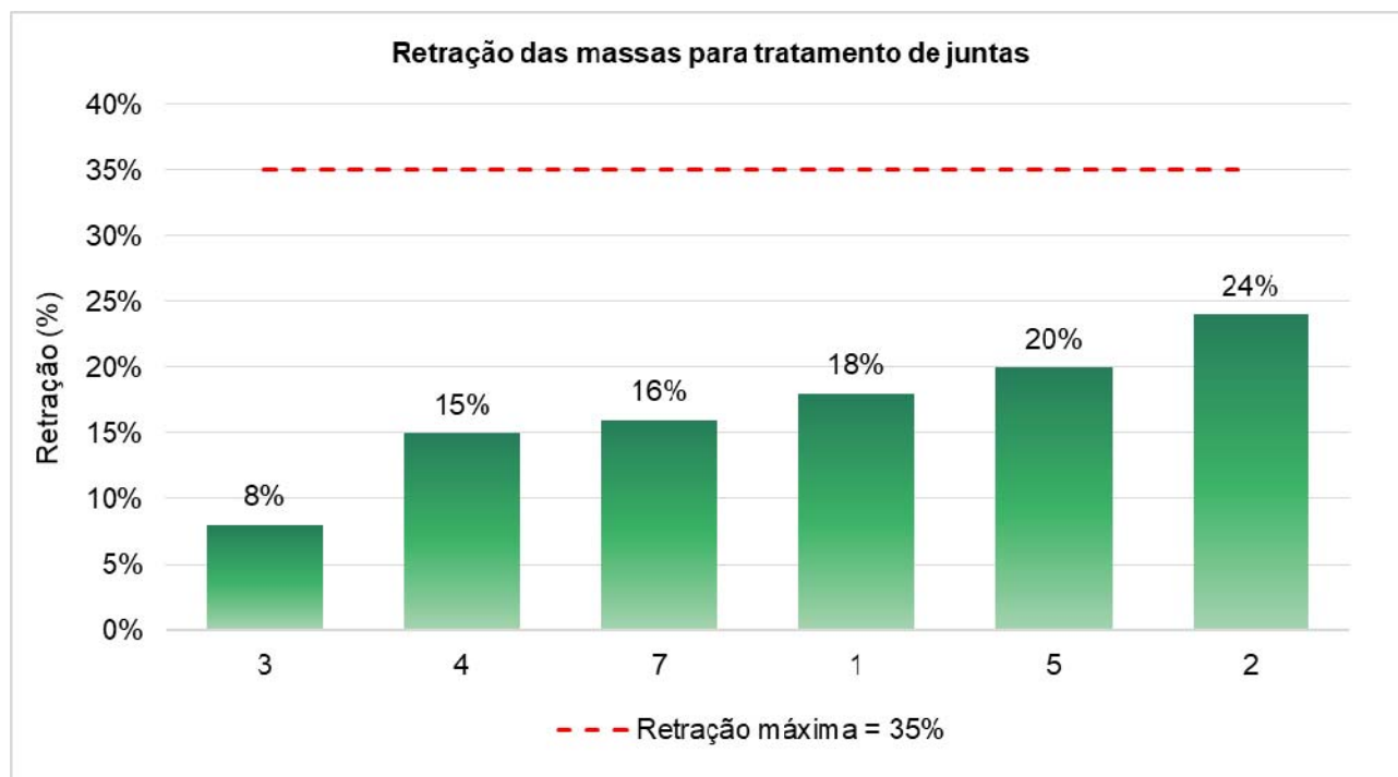
Figura 27 – Resultados da verificação da retração das amostras de massa para tratamento de juntas avaliadas (empresas participantes e marca acompanhada)
