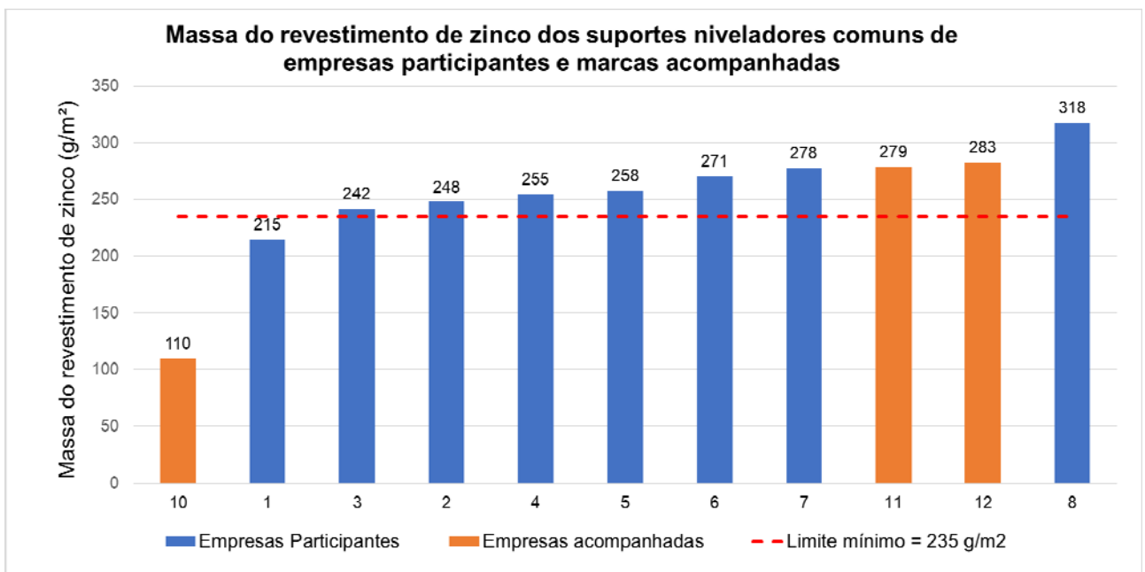
Figura 25 – Resultados da determinação da massa de revestimento de zinco das amostras de suporte nivelador comum avaliadas de empresas participantes e marcas acompanhadas (resultados da determinação da massa média de revestimento de zinco das amostras)
